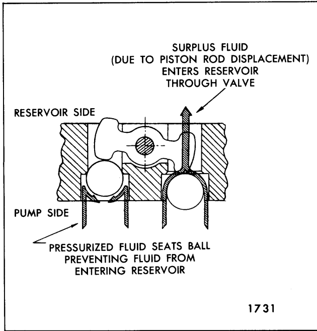
Fig. 13-62—Fluid Control Valve
